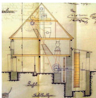
Severovýchodní průčelí mlýna, počátek 20. století a příčný řez mlýnem, 1897. Ve spodní mlýnici paleční kolo a převody, v horní mlýnici válcová mlecí stolice, v podkroví hranolový vysévač, v podstřeší triér a tarár
